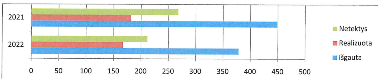
1 pav. UAB „Pagėgių komunalinis ūkis“ 2021-2022 m. vandens gavyba, realizacija, netektys, tūkst.m 3
